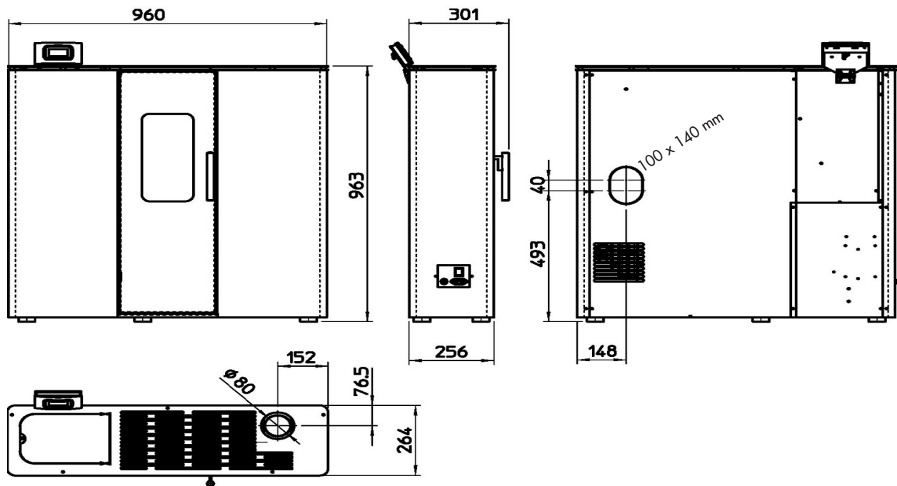
Abb. 2b: Geräteabmessungen (alle Maßangaben in mm)
